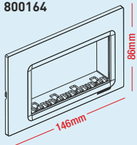
4 module 800164
