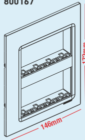
8 module (Vertical) 800167
