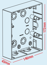
8 module (Vertical) 800187
