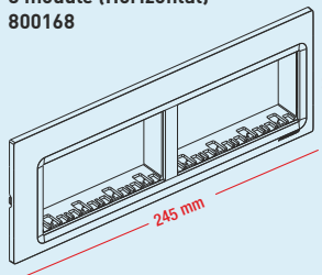
8 module (Horizontal) 800168
